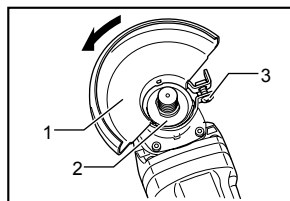
1. Protector (guarda) de disco 2. Caja de rodamientos 3. Tornillo
