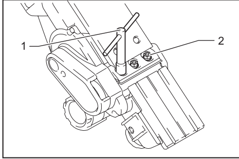
► 1. Llave de bujías 2. Perno de instalación
