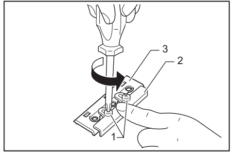
► 1. Tornillo 2. Placa de ajuste 3. Placa de fijación
