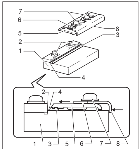
► 1. Calibrador de cuchillas 2. Borde interno del calibrador de cuchillas 3. Cuchilla del cepillo 4. Borde de la cuchilla (de la minicuchilla del cepillo) 5. Placa de fijación 6. Placa de ajuste 7. Tornillo 8. Pie
